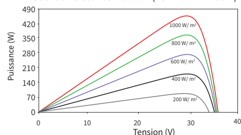
Courbe Puissance-Tension (48HL4M-DB 460W)
